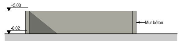
FACADE EST
