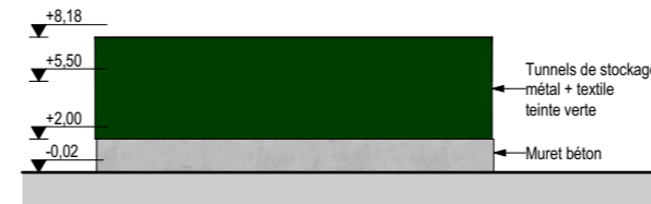
FACADE NORD
