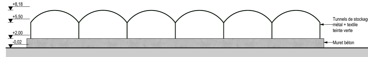
FACADE OUEST
